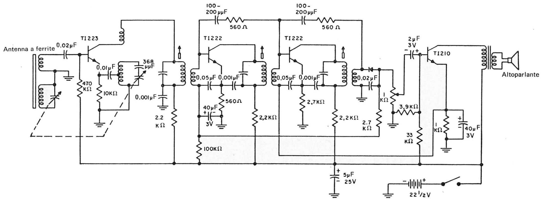
Figura 18.4. - Schema elettrico del radiorecettore tascabile Regency Mod. TR-1.
